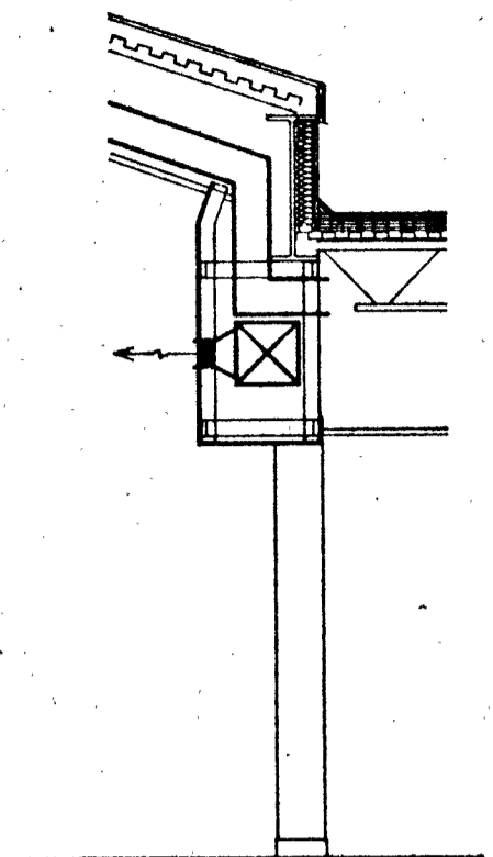
SECTION A-M4 (SCALE: 1/4"=1'-0")
